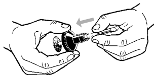
Oberes Sieb mit Hilfe des Reinigungspinsels herausdrücken
