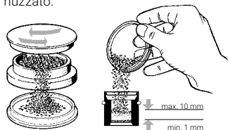
Riempire il Contenitore
